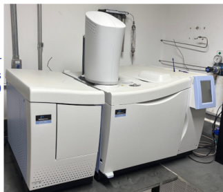
PERKINELMER – Clarus 600T Cromatógrafo Gasoso acoplado à Espectrometria de Massas Gas Chromatograph–Mass Spectrometer (GC-MS)
