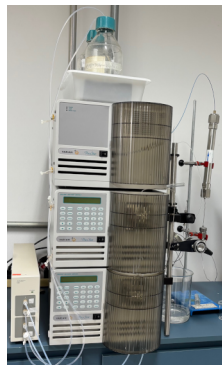
VARIAN – ProStar 210 / PrepStar 218 Cromatógrafo Líquido de Alta Eficiência Preparativo High-Performance Liquid Chromatograph (HPLC)
